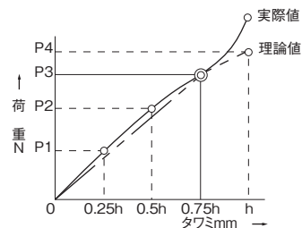
さらばねの荷重とタワミの関係
