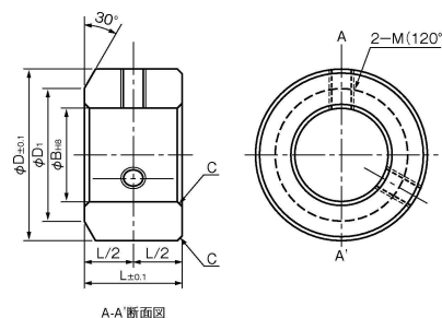
A-A 断面図
