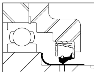
標準リップシールの 使用例
