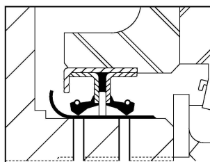
複合リップシールの 使用例
