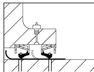
2個のスリーブを使 い、一方のフランジ を取り去った使用例
